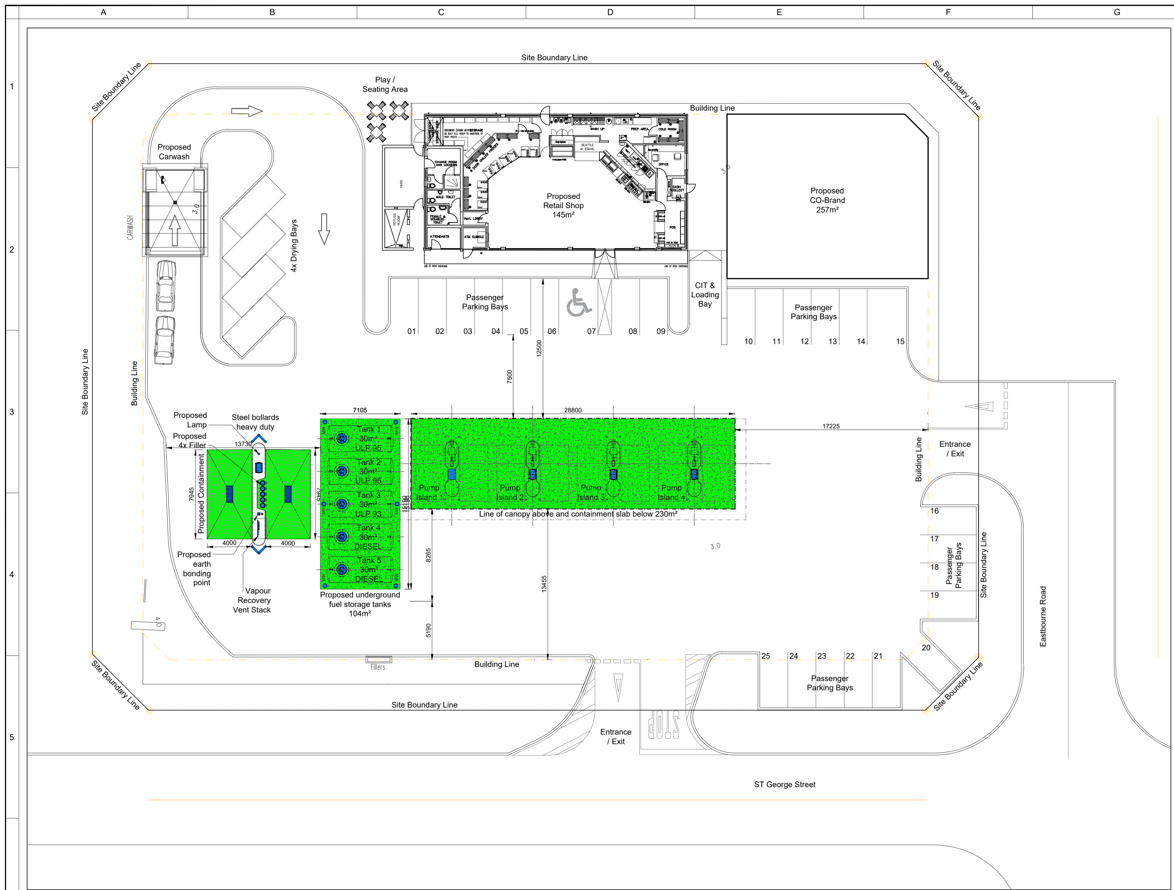
01 Site Plan 100 SCALE 1:200
